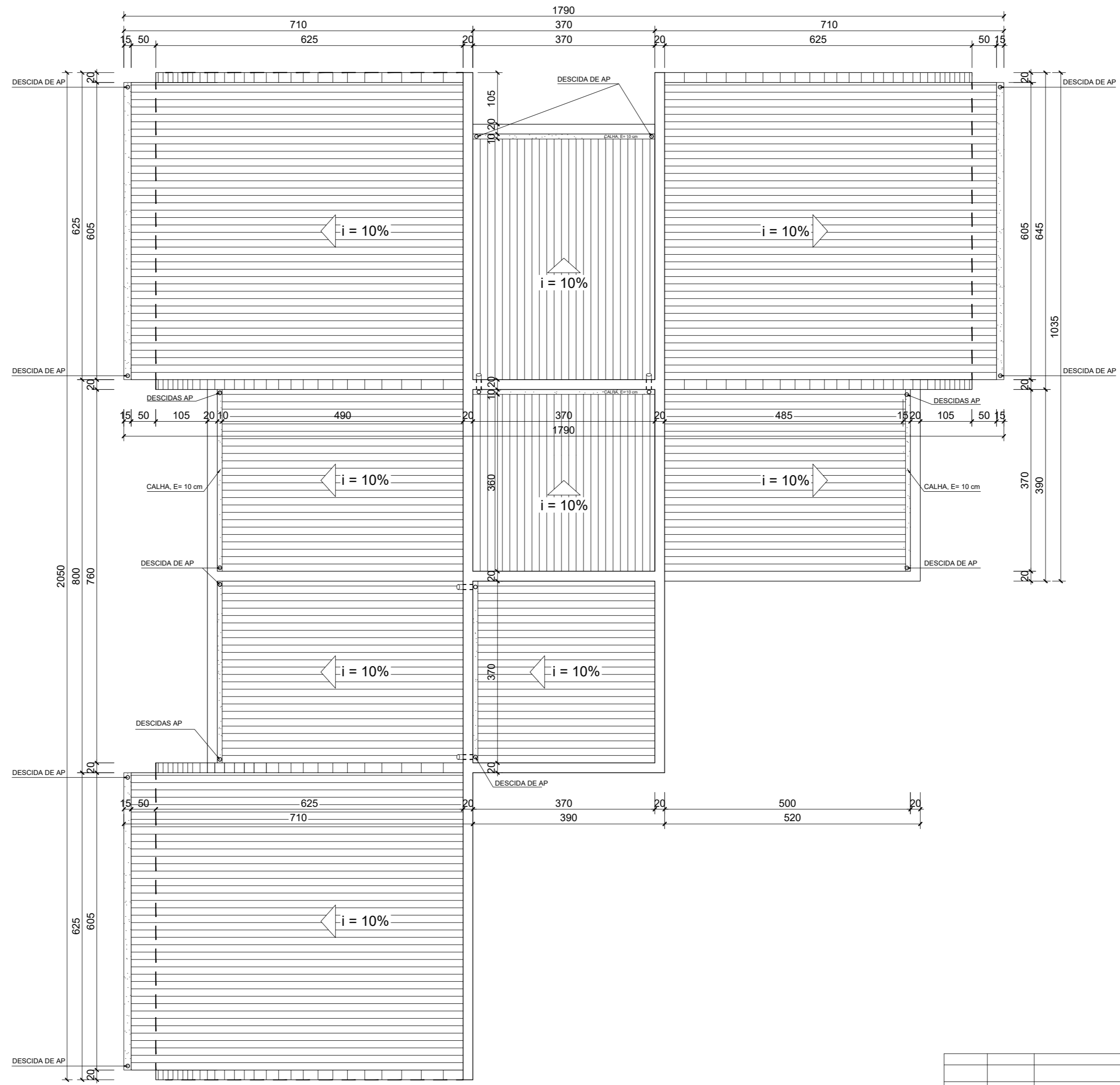
DIAGRAMA DE COBERTURA ESCALA 1/100
